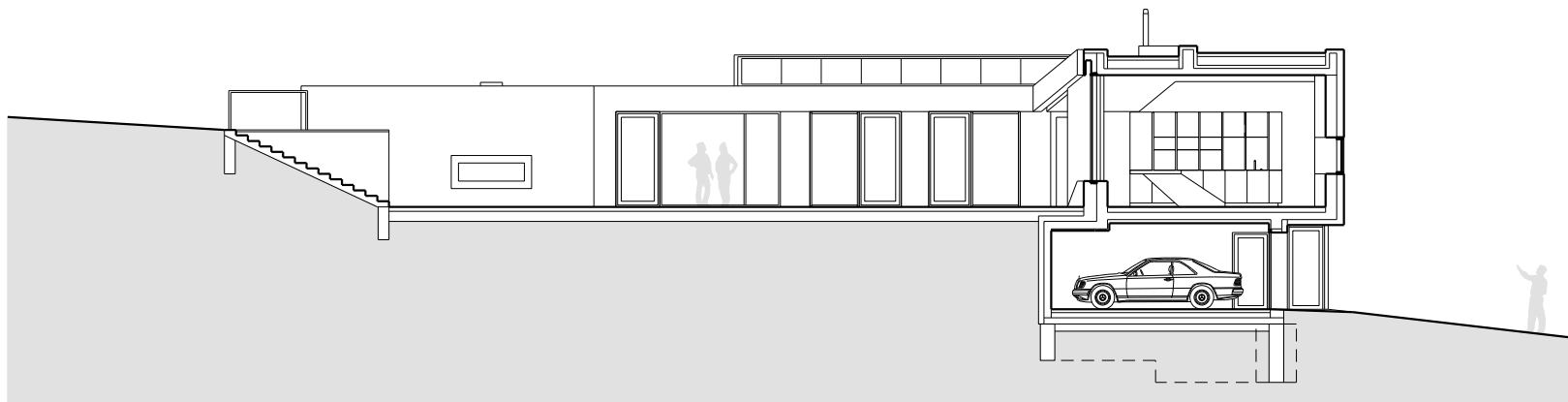
rez pozdĺžny
