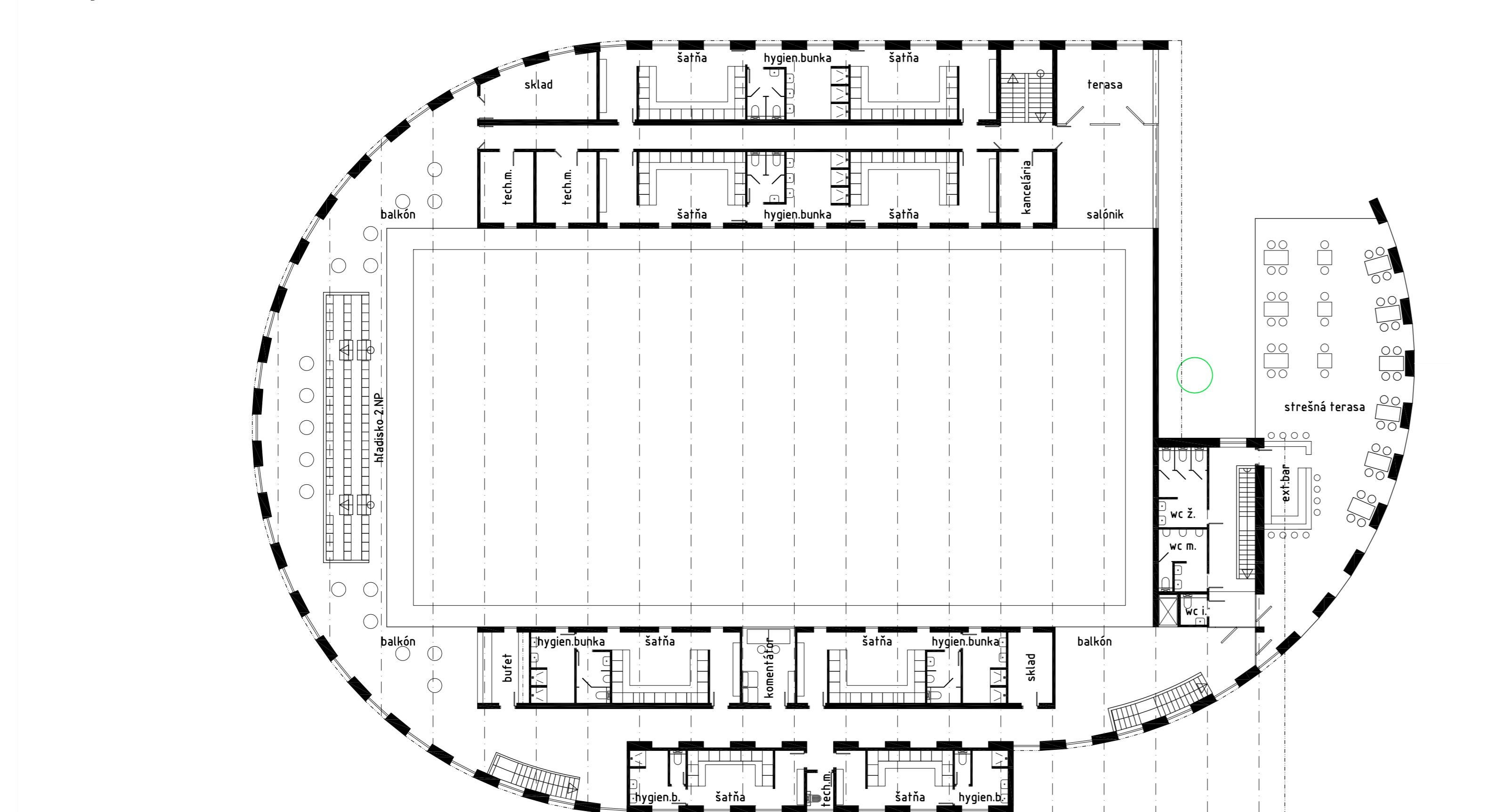
Pôdorys 2.NP
