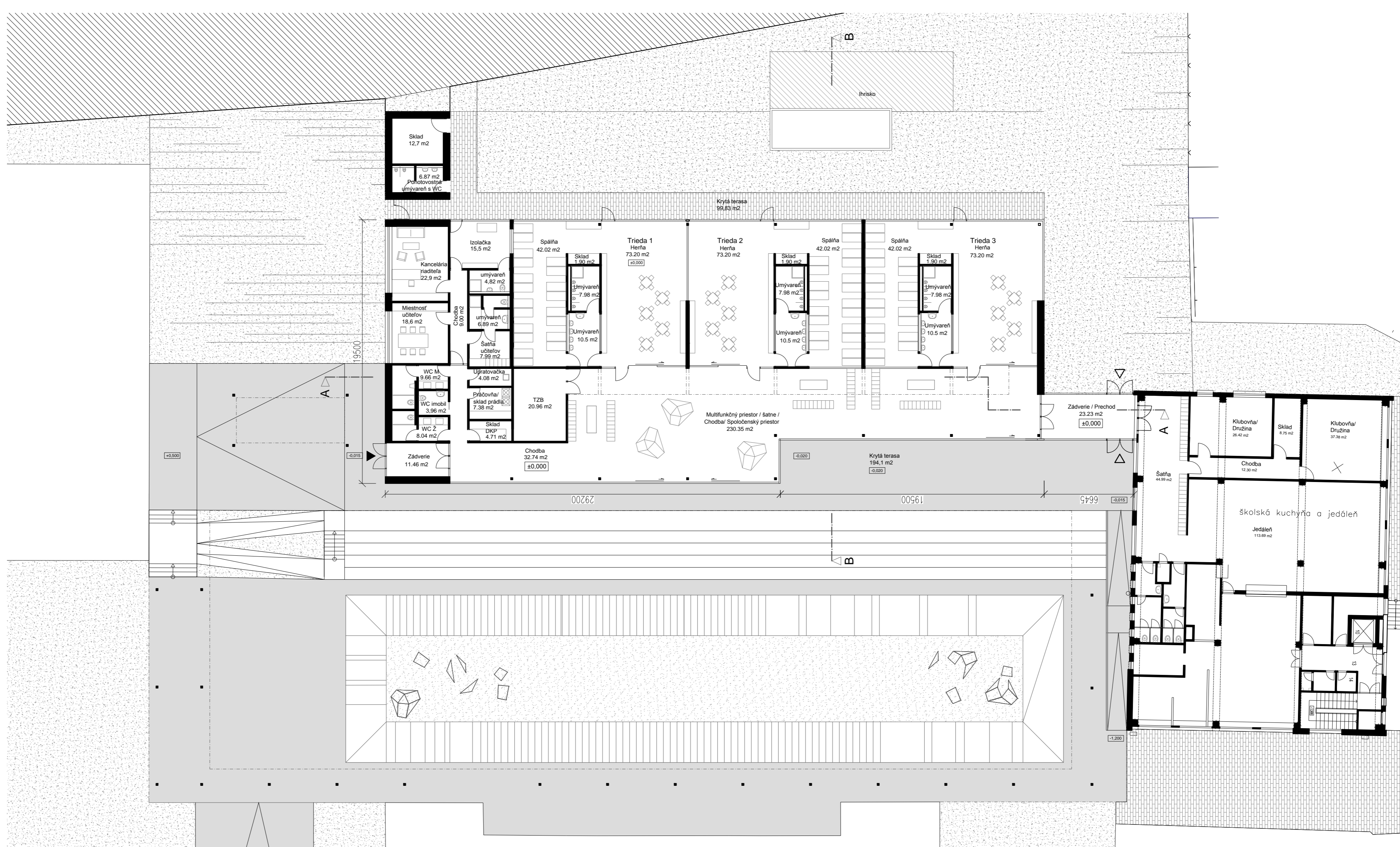
PÓDORYS 1.NP M 1:200
