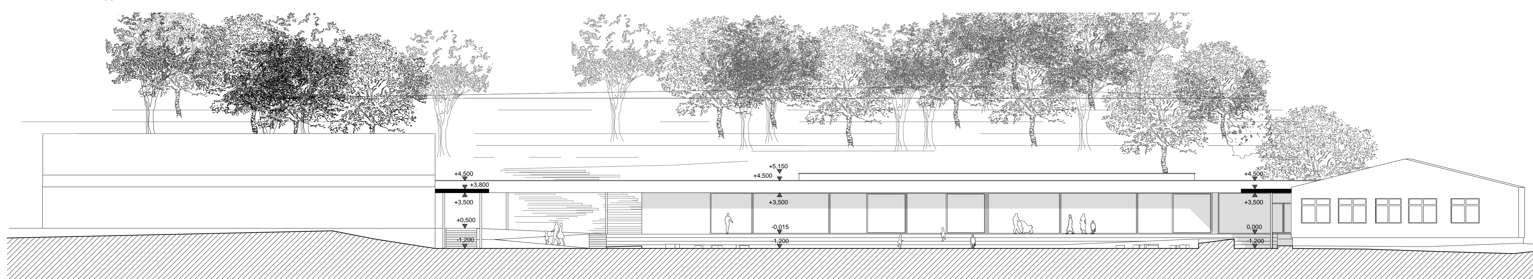
POHĽAD SEVEROZÁPADNÝ M 1:200
