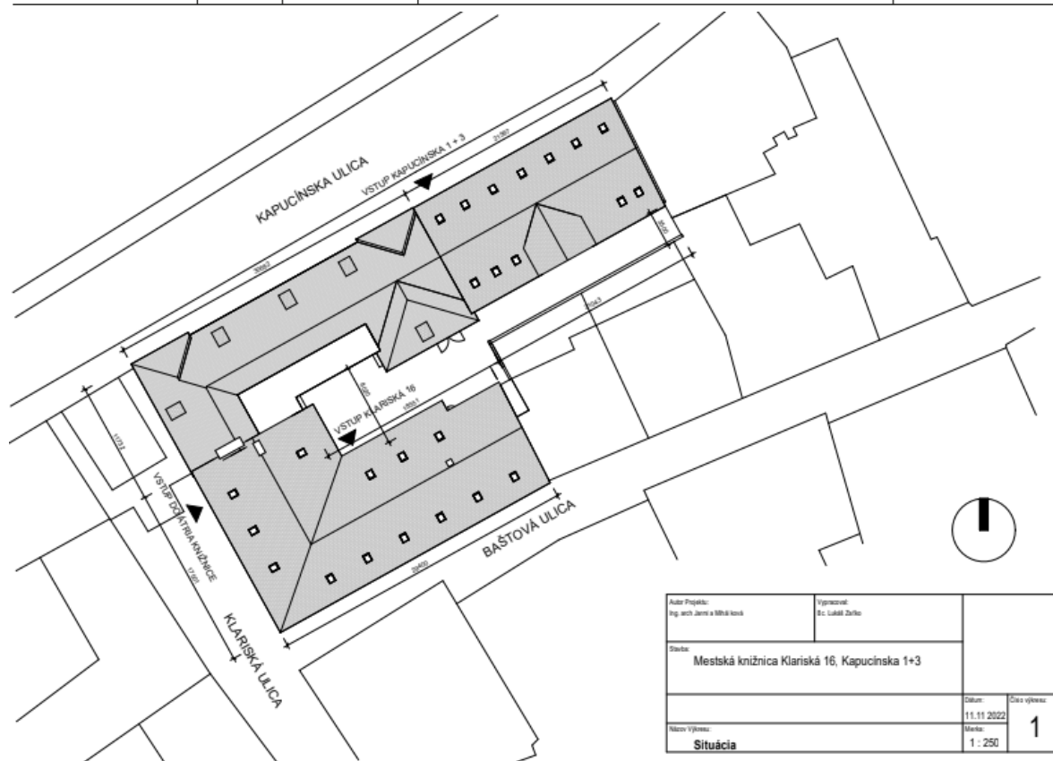
Obr. č. 2 Situačný náčrt objektov Kapucínska, Klariská
