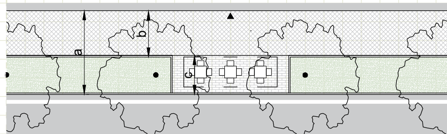
Schémy znázorňujú minimálne parametre pre umiestňovanie mobiliáru a terás ako súčasť chodníka s výsadbovými plochami.
