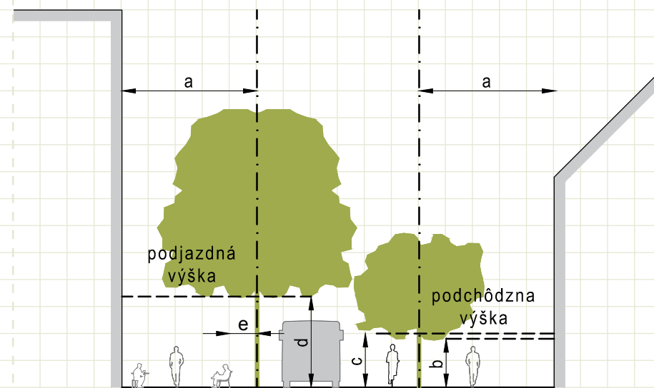
Schéma znázorňujúca optimálne parametre vzdialenosti výsadby v rámci spevnených plôch v uličnom profile.
